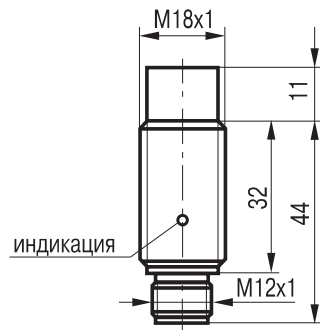
Габаритный чертёж
