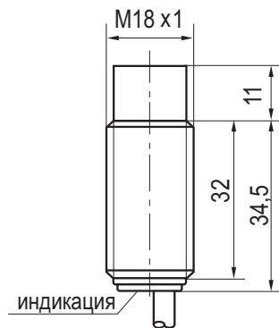
Габаритный чертеж
