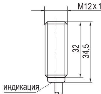
Габаритный чертеж
