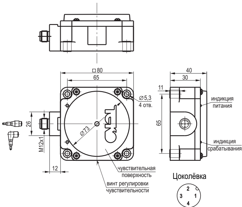
Габаритный чертеж
