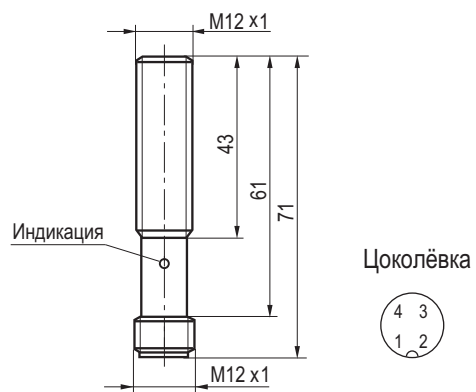
Габаритный чертеж
