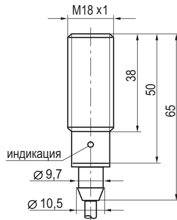
Габаритный чертеж
