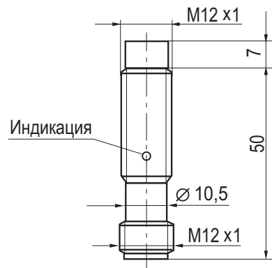
Габаритный чертеж
