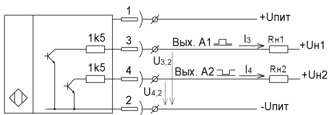
Схема подключения
