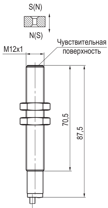
Габаритный чертеж
