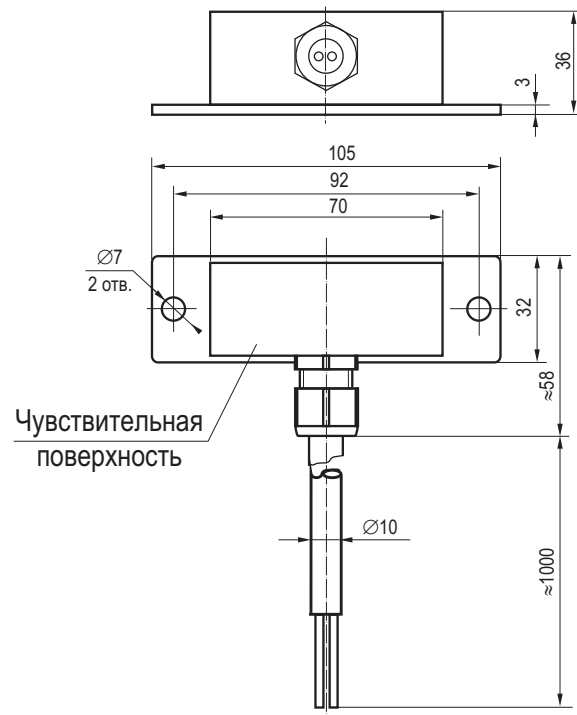
Габаритный чертеж
