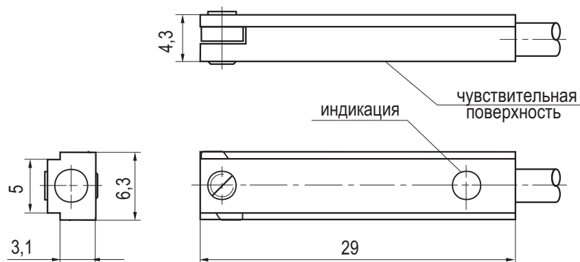
Габаритный чертеж
