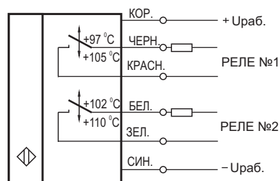
Схема подключения
