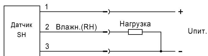
Схема подключения
