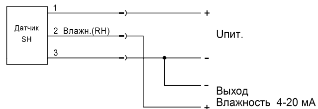
Схема подключения
