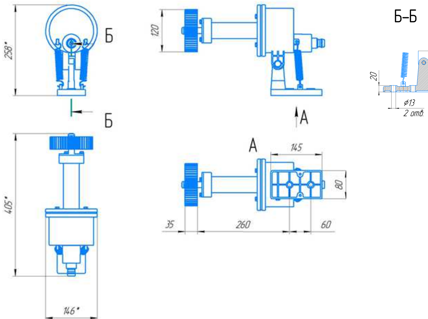
Габаритный чертеж
