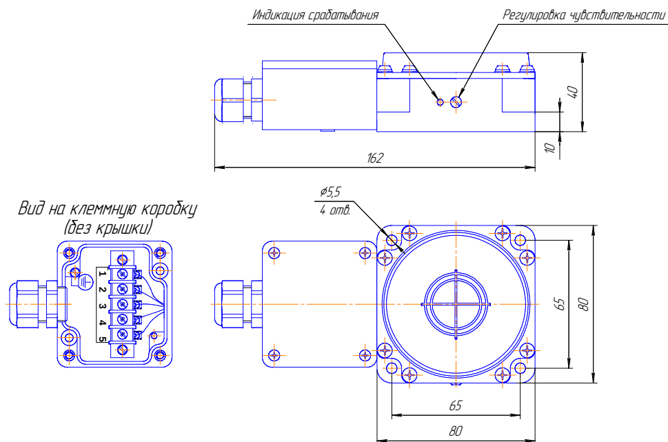
Габаритный чертеж
