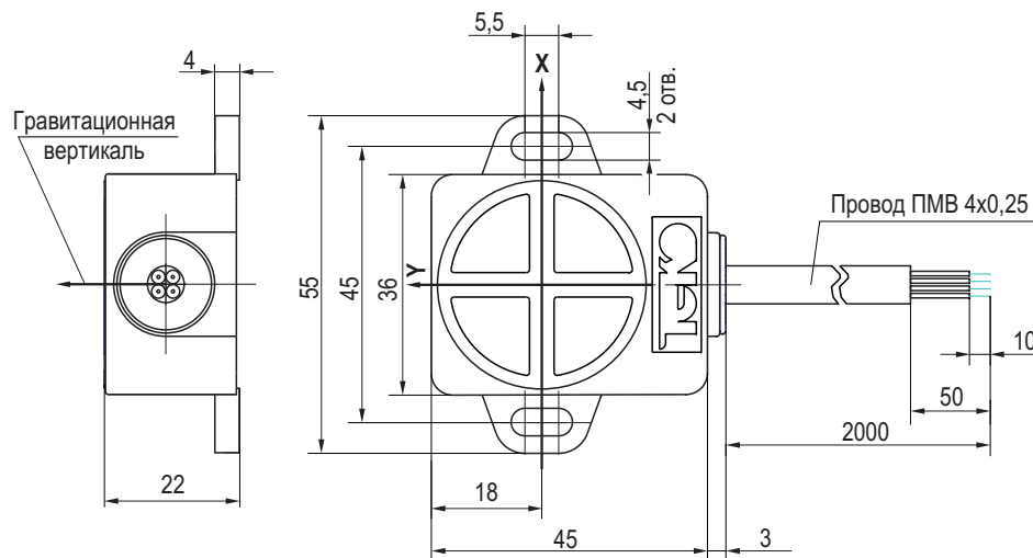
Габаритный чертеж
