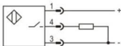
PNP NO
