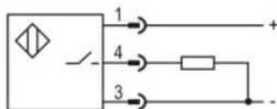
PNP NO
