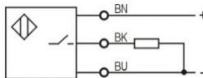
PNP NO
