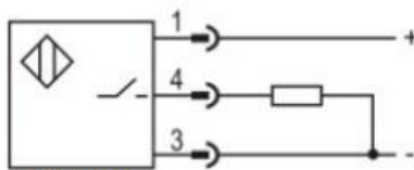
PNP NO
