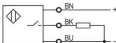
PNP NO
