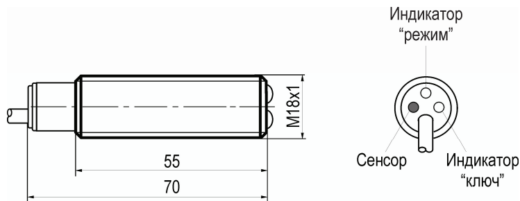
Рисунок 1 - Габаритный чертёж
