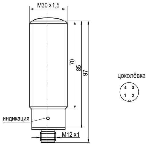
Габаритный чертеж.
