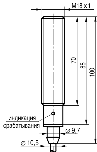
Габаритный чертеж.
