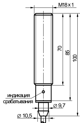
Габаритный чертеж.
