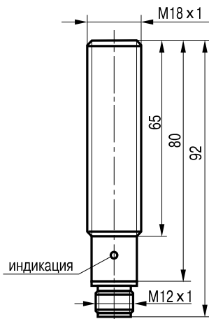
Габаритный чертеж.
