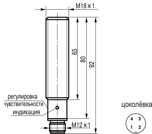
Габаритный чертеж.
