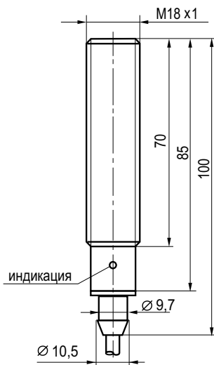
Габаритный чертеж.
