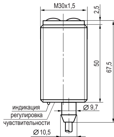
Габаритный чертеж.
