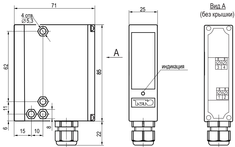
Габаритный чертеж.
