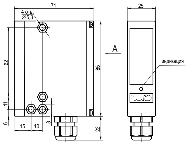
Габаритный чертеж.
