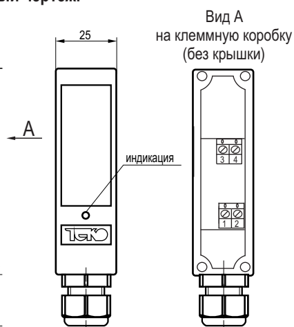
Габаритный чертеж.
