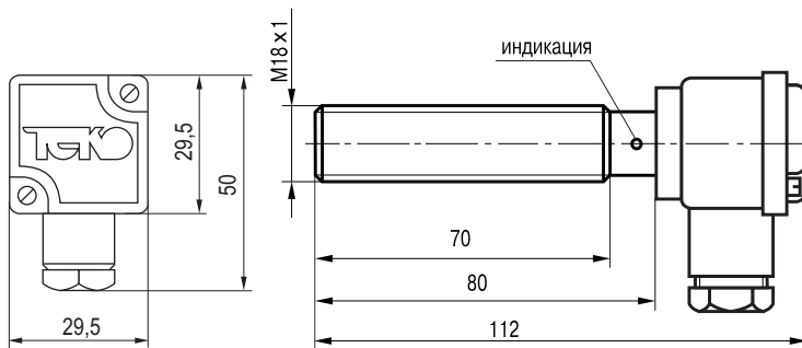
Габаритный чертеж
