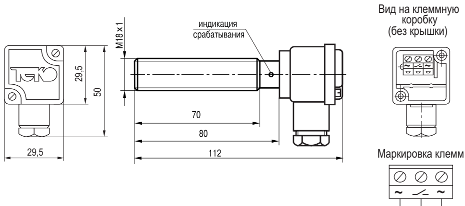
Габаритный чертеж
