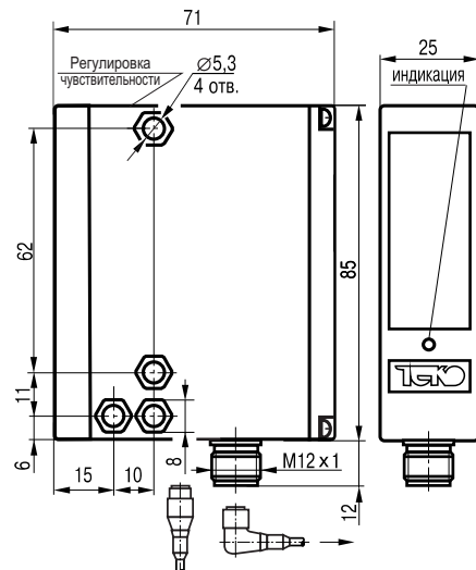
Габаритный чертеж
