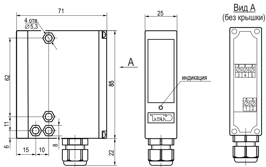
Габаритный чертеж
