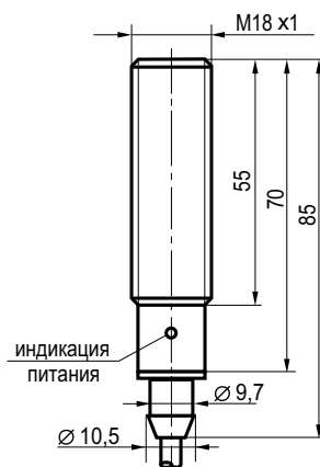
Габаритный чертеж
