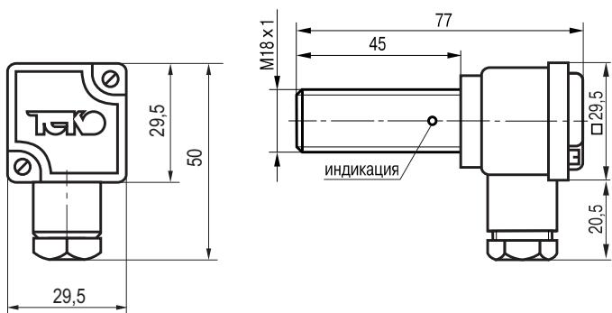
Габаритный чертеж
