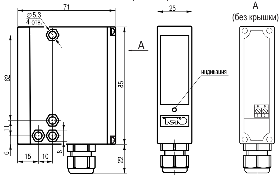
Габаритный чертеж
