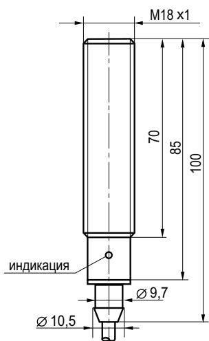
Габаритный чертеж
