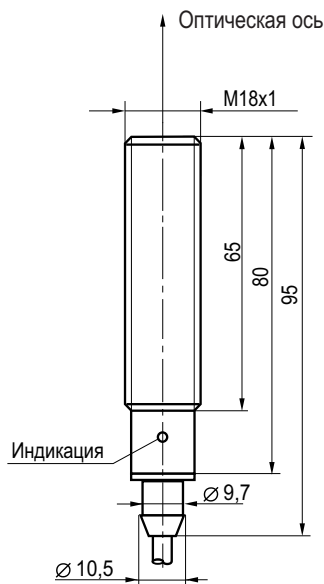
Габаритный чертеж
