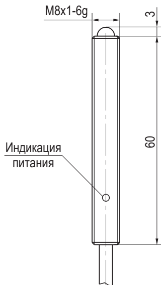
Габаритный чертеж
