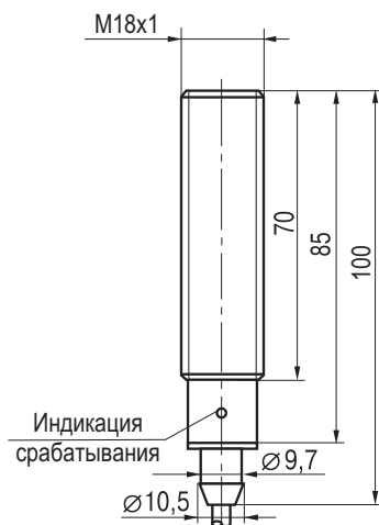
Габаритный чертеж
