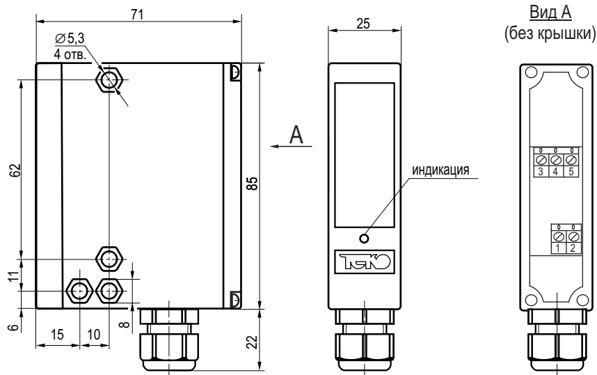
Габаритный чертеж
