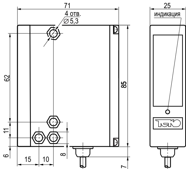
Габаритный чертеж
