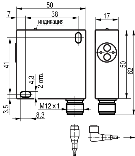
Габаритный чертеж
