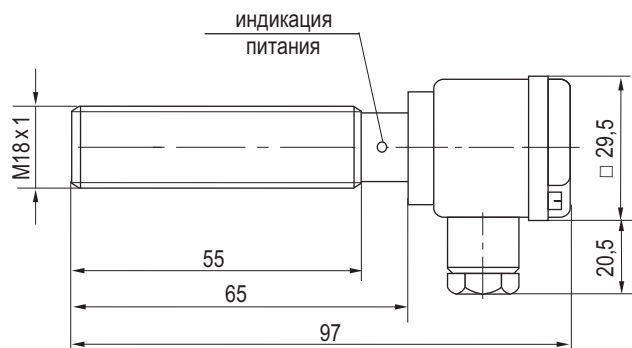
Габаритный чертеж
