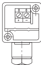
Вид на клеммную коробку (без крышки)
