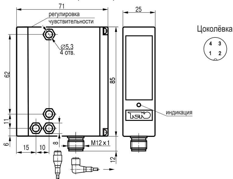
Габаритный чертеж.
