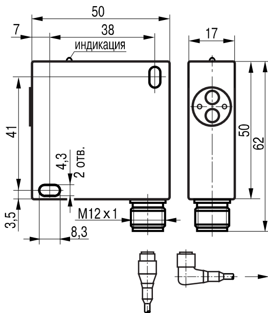
Габаритный чертеж
